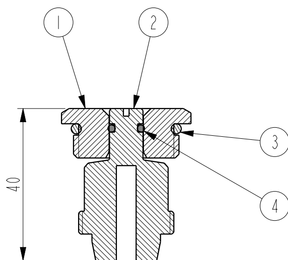
断面 A-A
