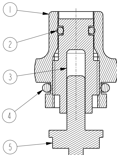
断面 A-A
