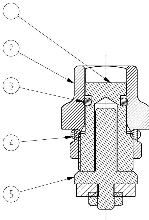
断面 A-A
