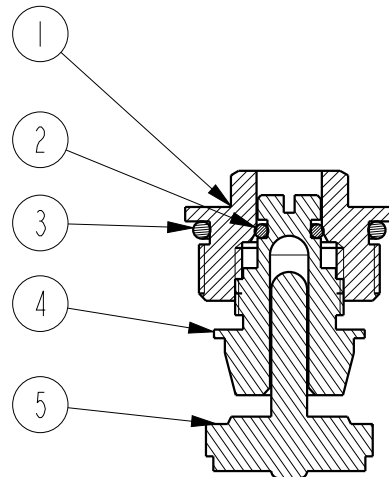
断面 A-A
