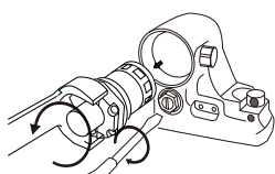
マイナスドライバで止水し立ち カラン締めで電磁弁を外す
