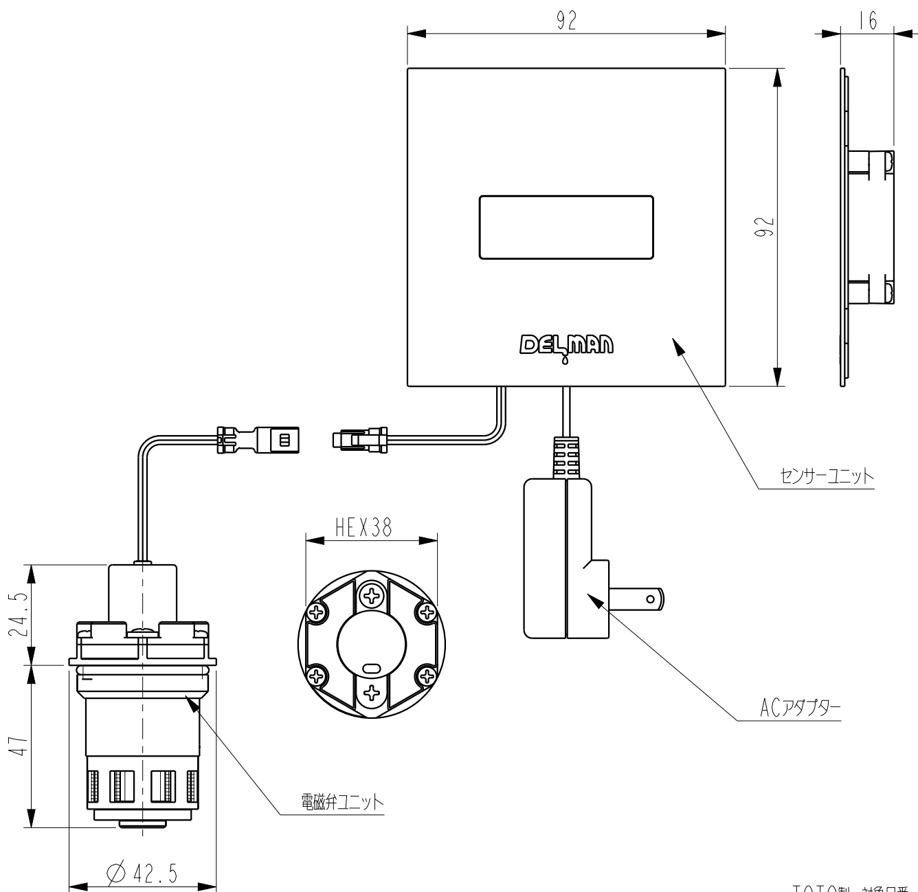
AC止水パーツ
