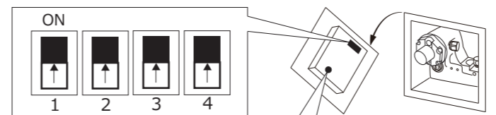
ディップスイッチ ※出荷時全て ON (上) 変更後、手動スイッチ長押し
