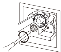
マイナスドライバで止水し立ちカラン締めで電磁弁を外す
