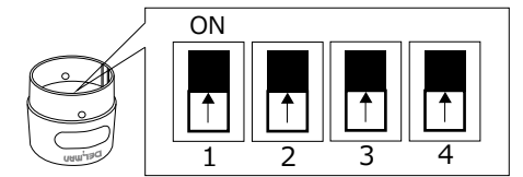
ディップスイッチ部 拡大図 ※出荷時は全てON (上)
